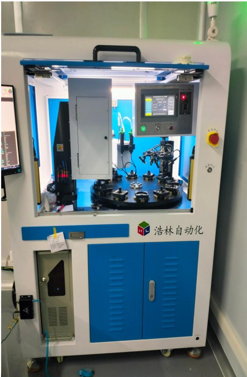
自动调焦机
