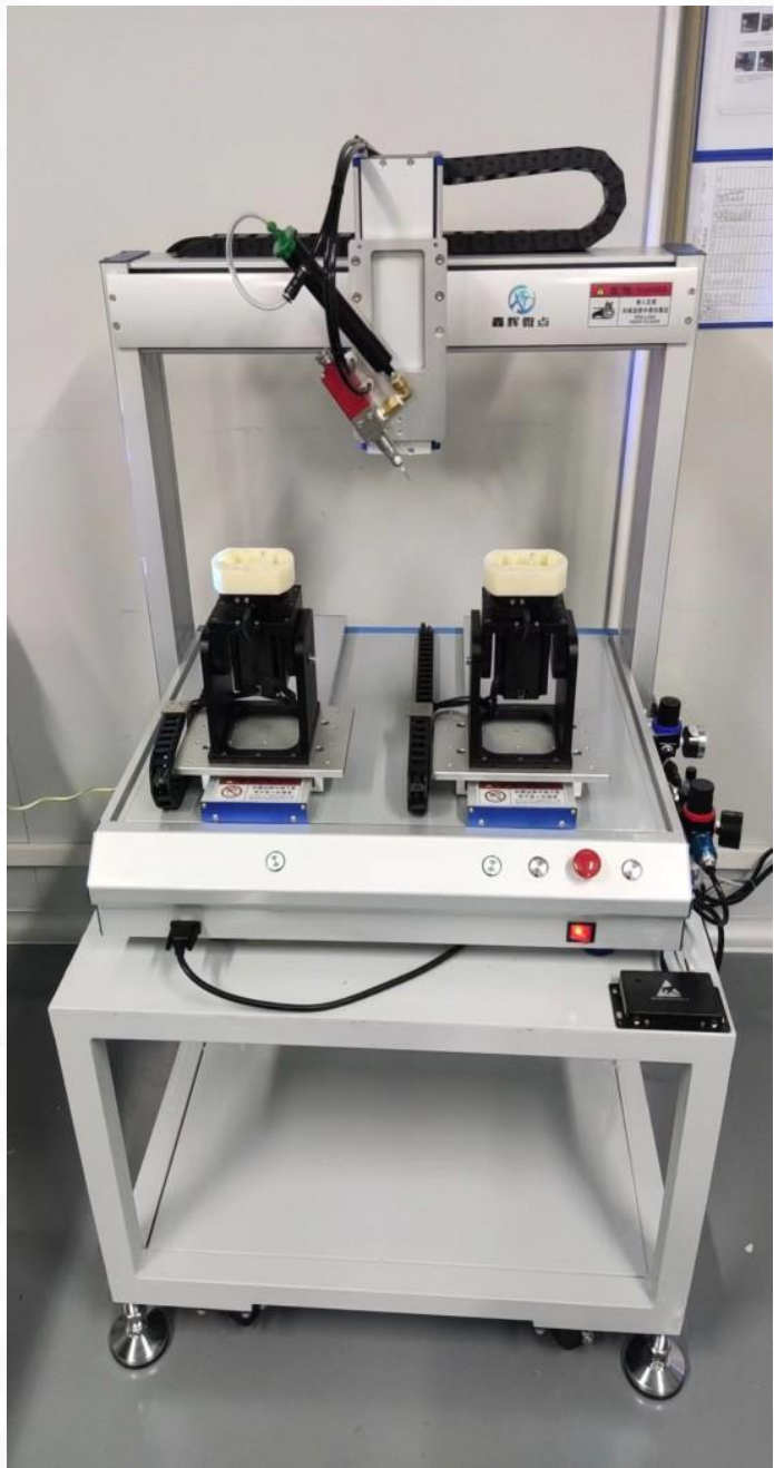
自动点胶机
