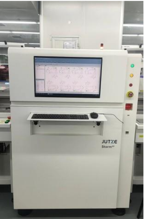
SPI锡膏印刷检测机
